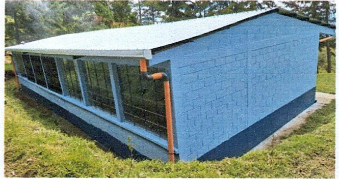
Foto 2: ÁREA DE LA PARTE DE ATRÁS DONDE SE REALIZÓ EL MEJORAMIENTO DE TECHO, MANTENIMIENTO DE COSTANERAS Y MEJORAMIENTO DE CANALETAS CON SU RESPECTIVA CAIDA DE AGUA FINALIZADO.
